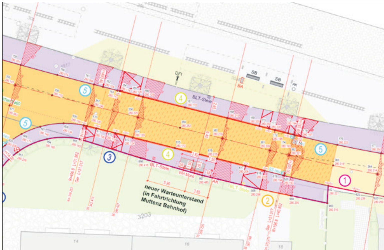
Ausschnitt aus Projektplan, BehiG-konforme Bushaltestelle FHNW vor den Liegenschaften Genossenschaftsstrasse 14/16 mit zusätzlichem Warteunterstand auf der südlichen Strassenseite.
